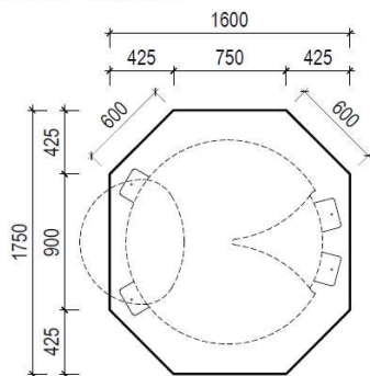
PŮDORYS ZÁKLADU
