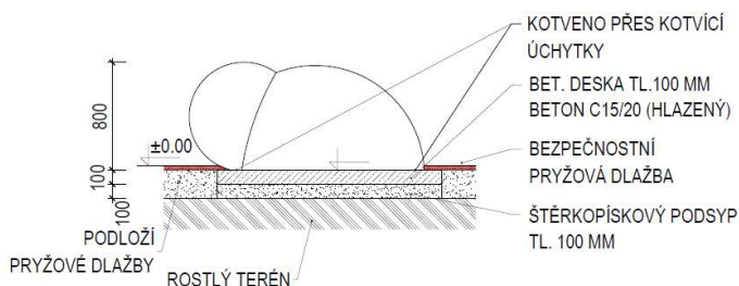
ŘEZ ZÁKLADEM
