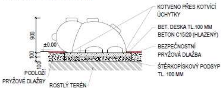
DOPADOVÁ PLOCHA - PRYŽOVÁ DLAŽBA
