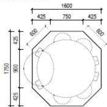
PŮDORYS ZÁKLADU
