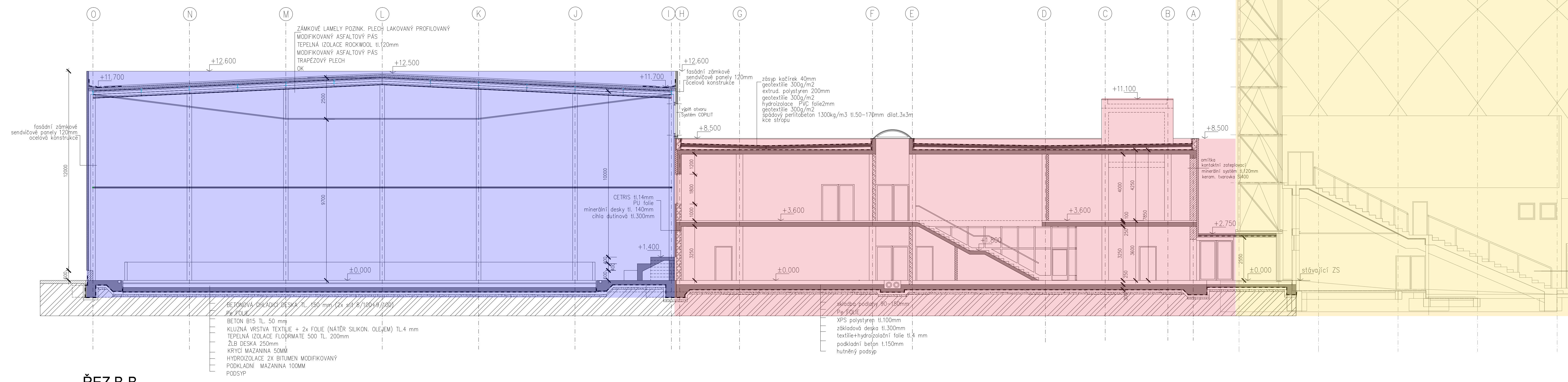
ŘEZ B-B
